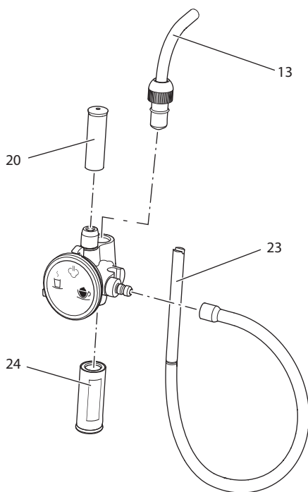
Рис. 17: Разборка капучинатора
